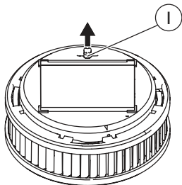
Abb. 8 Aktivierungstaste herausziehen
