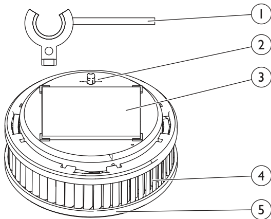
Abb. 1 Bedienelemente
